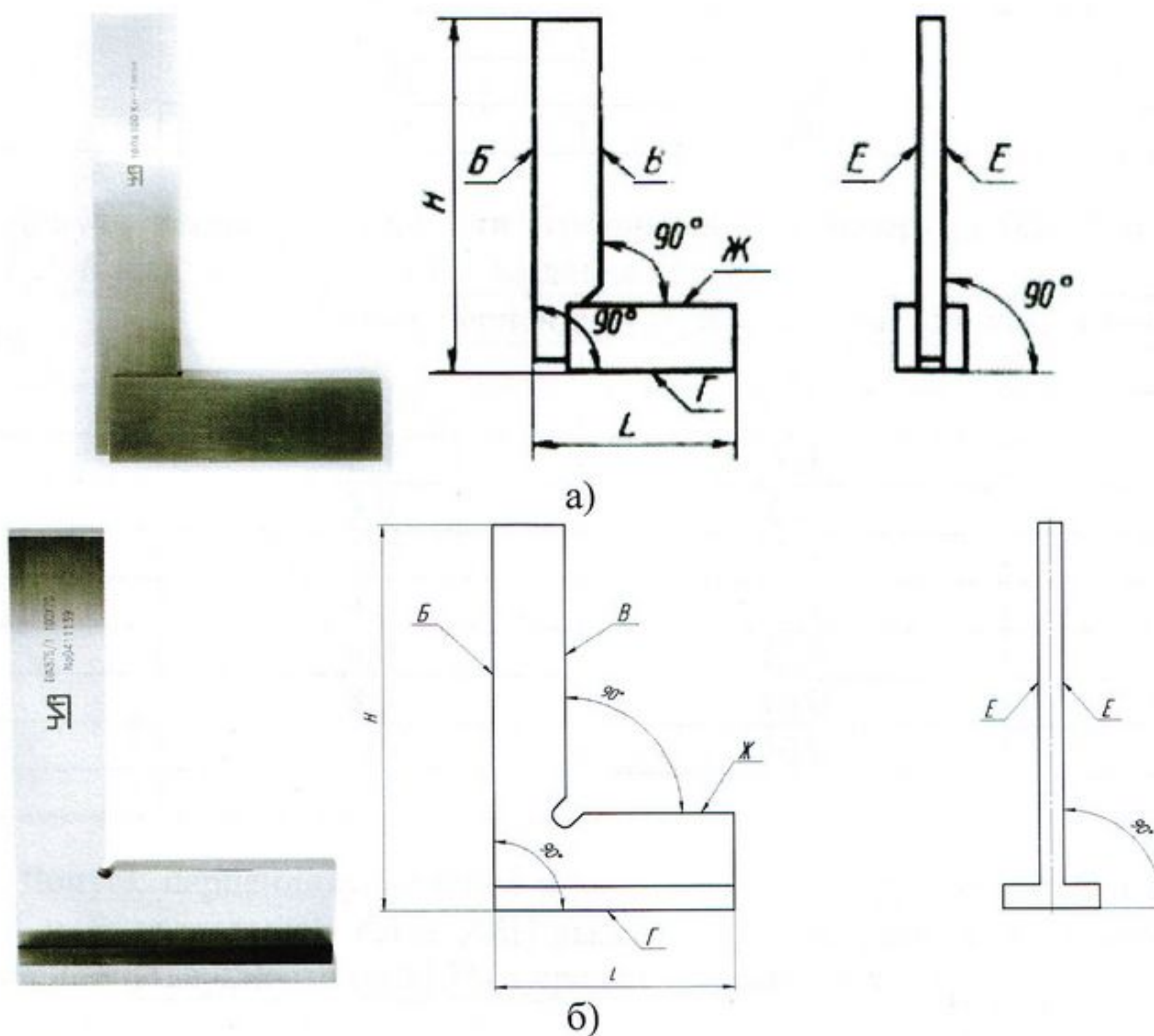
Рисунок 3 – Общий вид угольников УП, обозначение основных размеров и поверхностей
